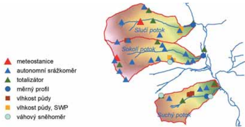
Obr. 2 Vybavení povodí měřicí technikou.
