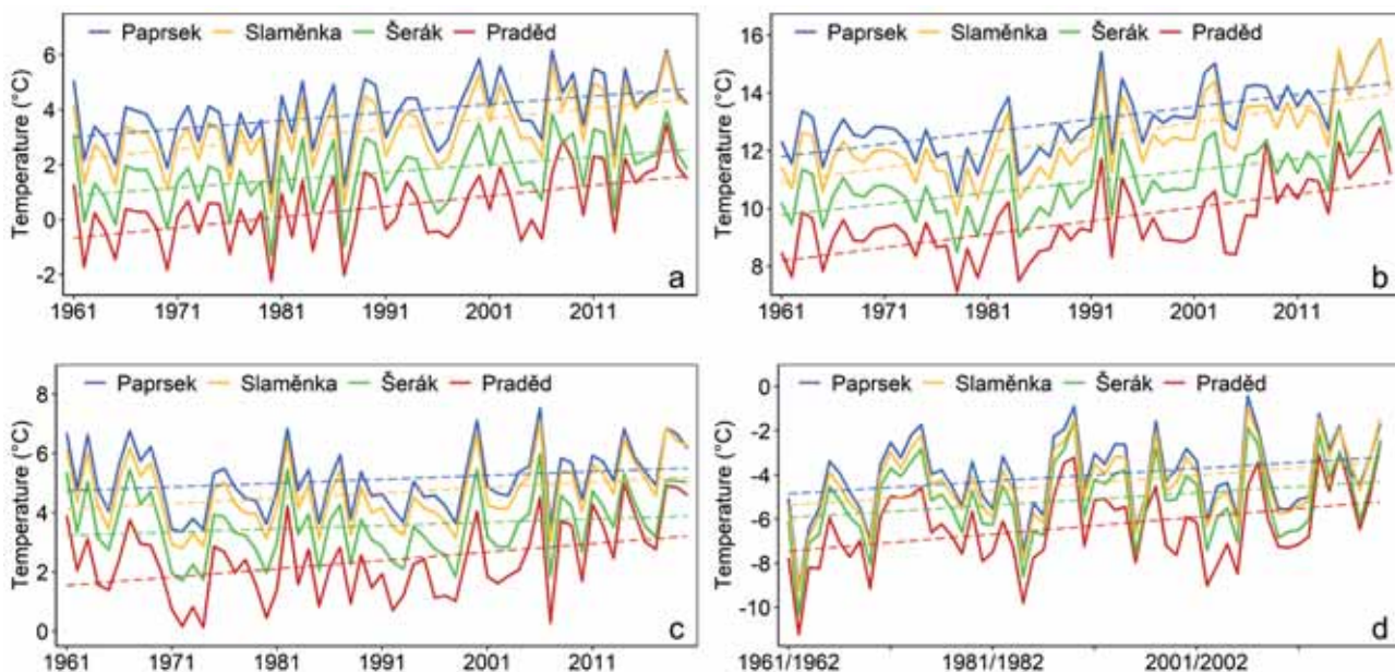
Obr. 2 Sezónní variabilita teploty vzduchu na meteorologických stanicích Paprspek, Praděd, Slaměnka a Šerák (a) na jaře, (b) v létě, (c) na podzim a (d) v zimě v období 1961–2020.
