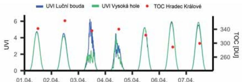
Obr. 4 Denní chod UVI na Luční boudě (modře) a na Vysoké holi (zeleně) 1.–7. dubna 2020 doplněný o průměrné denní množství ozonu (TOC, červeně).
