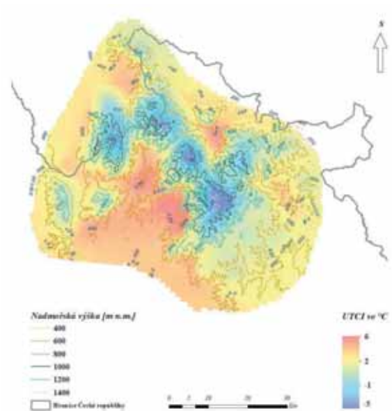
Obr. 2 Roční průměrné hodnoty UTCI a výškopis v oblasti Jeseníků.
