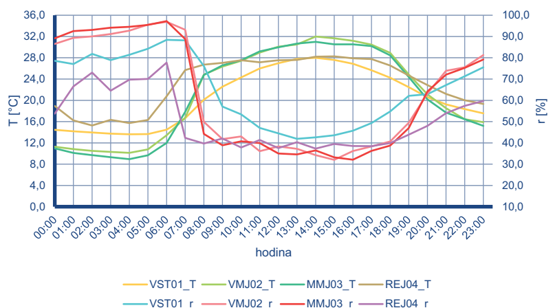
Obr. 2 Režim denní teploty vzduchu (T) a relativní vlhkosti vzduchu (r) na stanicích v NPR Rejvíz a osadě Rejvíz 20. 7. 2022. Zdroj: vlastní zpracování.
