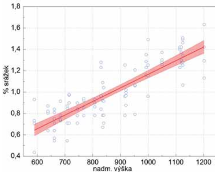
Obr. 3 Závislost relativního množství srážek (poměr aktuální hodnoty v měřícím bodě s průměrem za celá povodí) na nadmořské výšce v povodích Slučího, Sokolího a Suchého potoka (% srážek = -0,1072 + 0,0013 * x ; 0,95 Conf. Int.).
