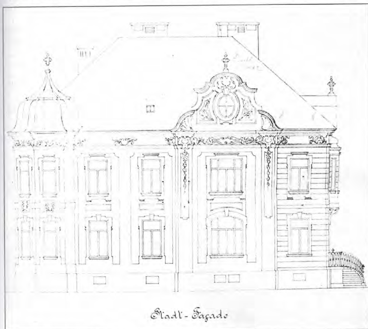
Regenhartova vila č.p. 62, technický výkres (SOKA Jeseník)
