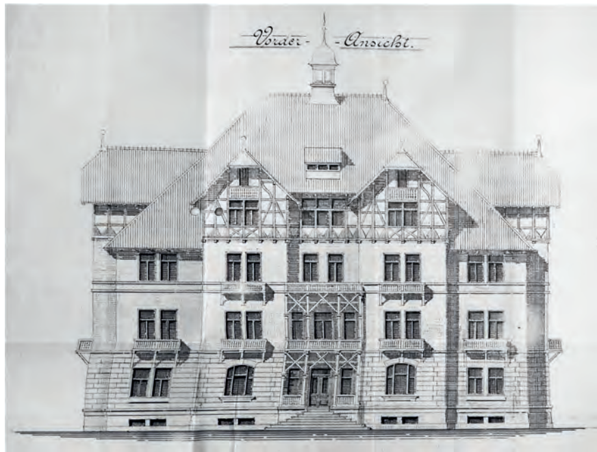
Obr. 4 Lipová-lázně, neprovedené rozšíření lázní o lázeňský dům Rochuse Schrotha, čelní pohled, 1906 (SOKA Jeseník, Místní národní výbor Dolní Lipová, nezpracované dodatky)
