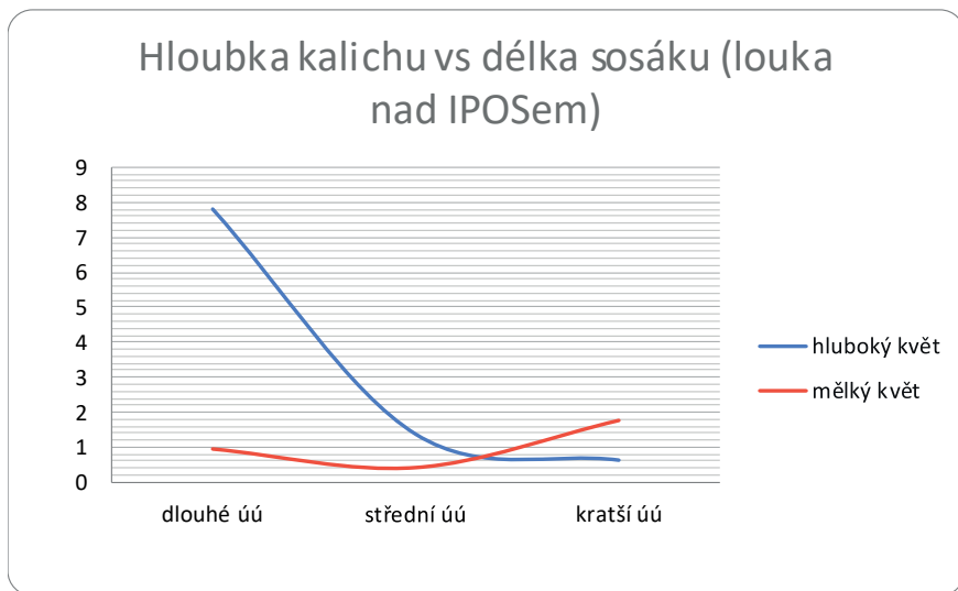
Grafy 3 a 4. Vztah hloubky kalichu a délky ústního ústrojí po normalizaci dat.
