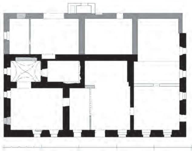
Obr. 2 Plán přízemí zámku po částečném zřícení zdíva. Plně značeno předpokládané zdivo nejstarší stavební fáze, tmavě šedě zdivo pozdějšího rozšíření budovy, světle šedě nejmladší konstrukce s přístavbou. Zaměření Ivo Stránský a Jiří Úlovec ve dnech 10. listopadu 2006 a 14. února 2008, měřítko po pěti metrech (kresba a úprava autor)
