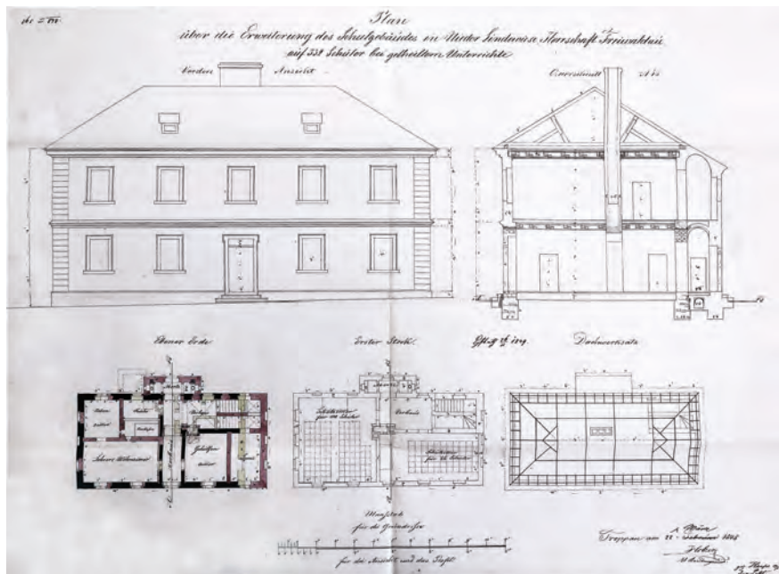
Obr. 2 Lipová-lázně, rozšíření školní budovy, 1848 (SOKA Jeseník, Okresní úřad Jeseník, inv. č. 773, karton 147)
